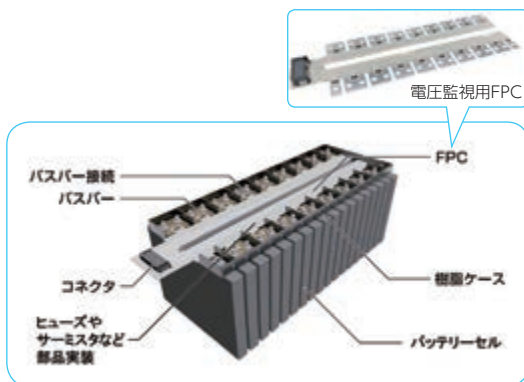
FPCを使用したリチウムイオン電池の電圧監視回路例
